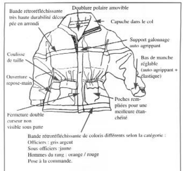
Dessin technique du Parka Microporeux
